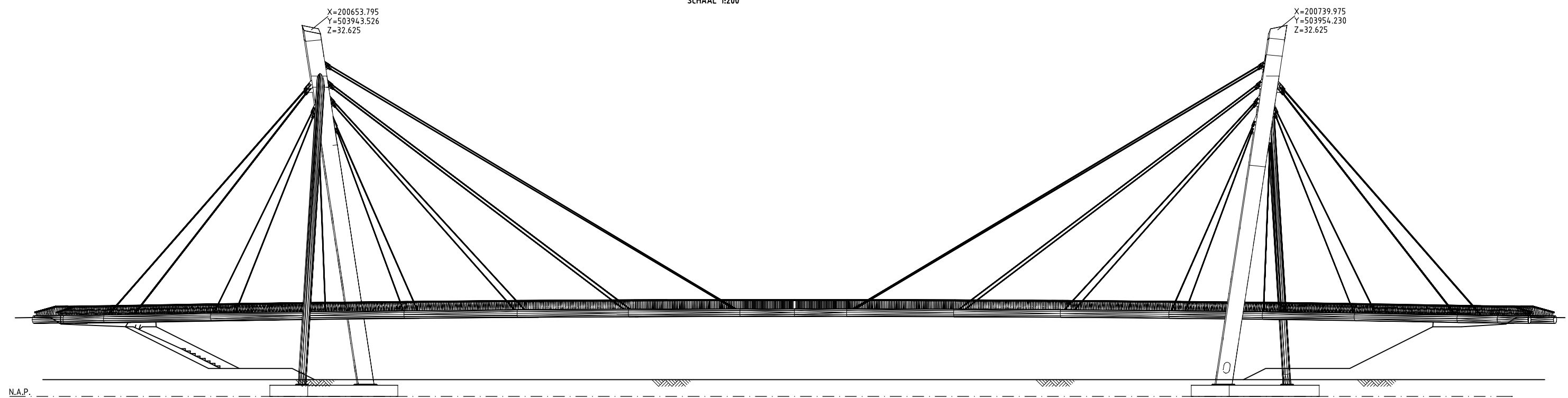
ZIJEAANZICHT SCHAAL 1:200
