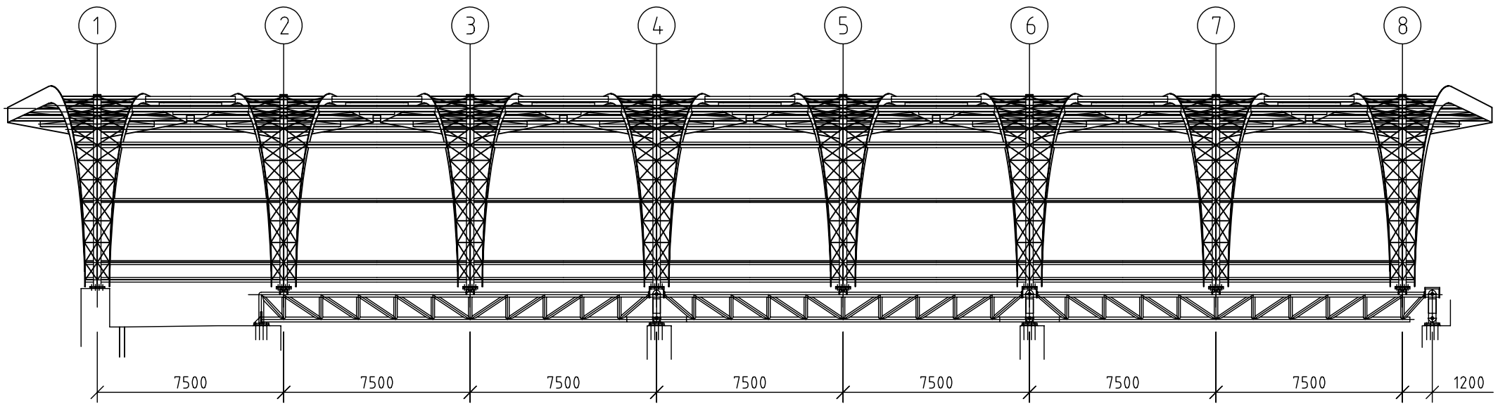
aanzicht staalconstructie (Noordzijde)
