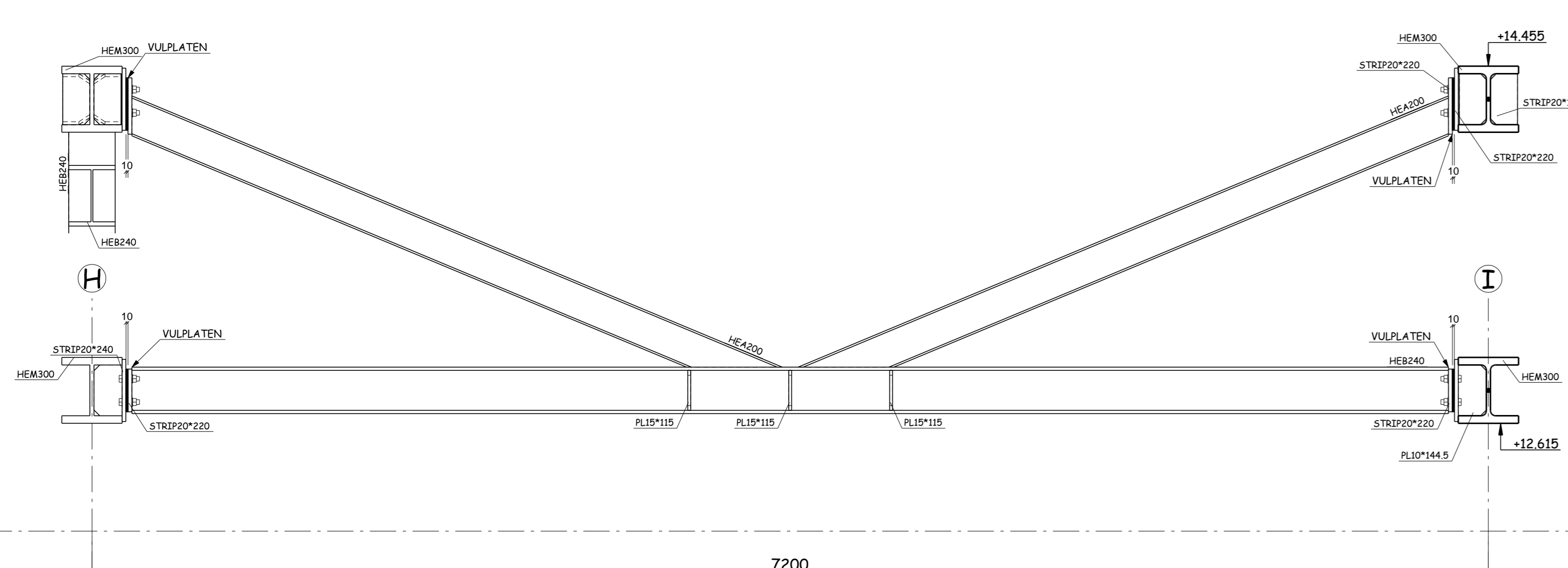
AANZICHT TUSSEN AS- 1 + 2
