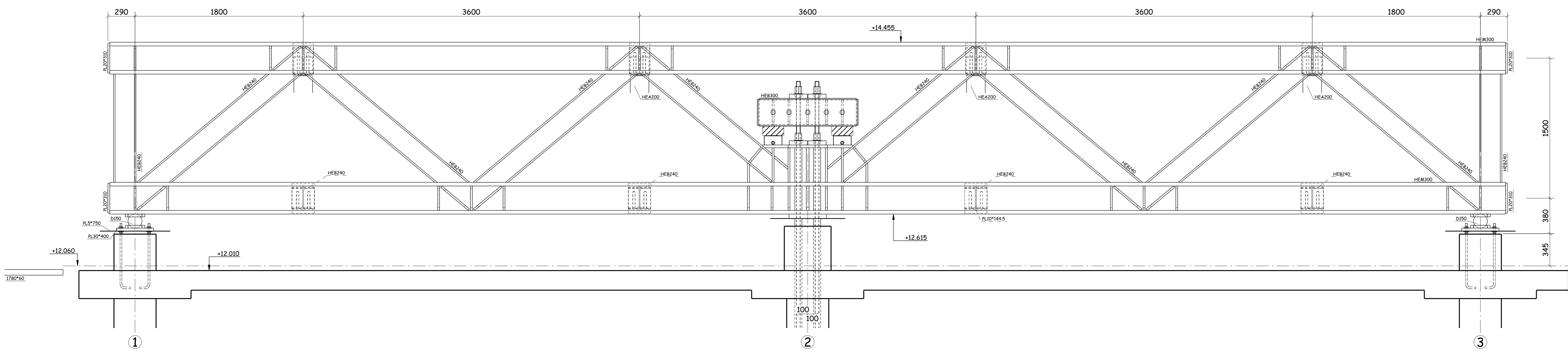
AANZICHT AS- H + I
