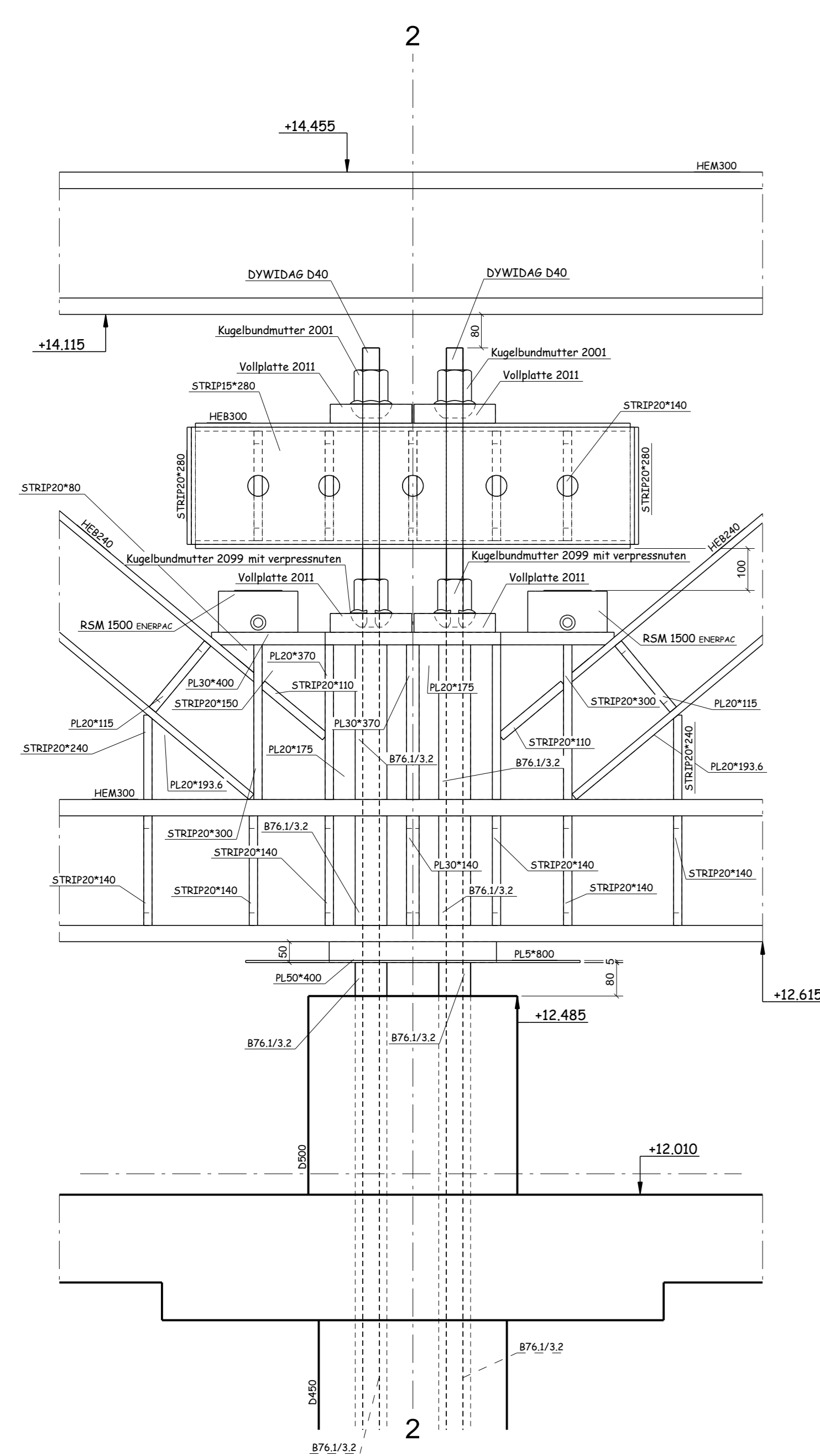
DETAIL VIJZELS
