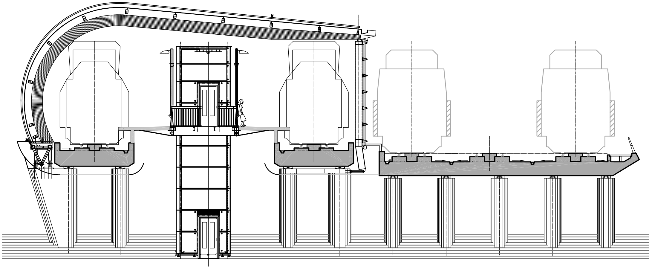
Doorsnede B-B
