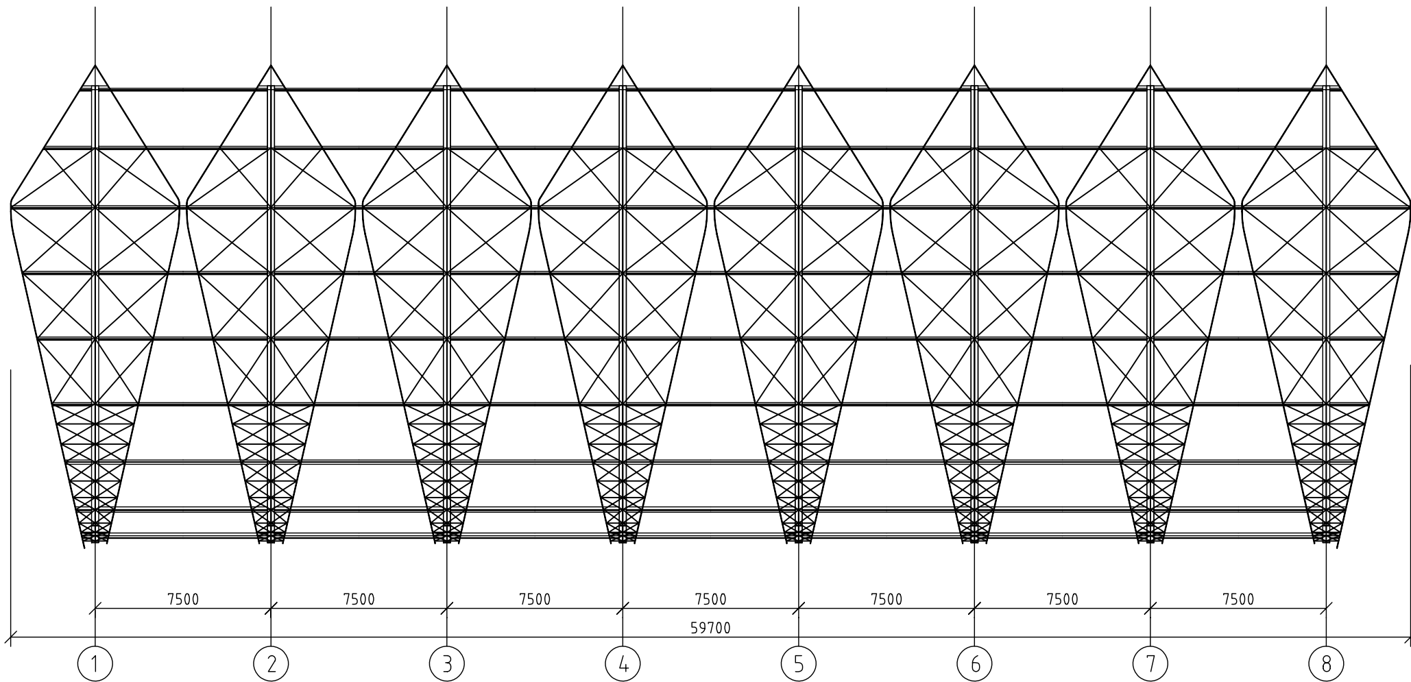
Bovenaanzicht staalconstructie
