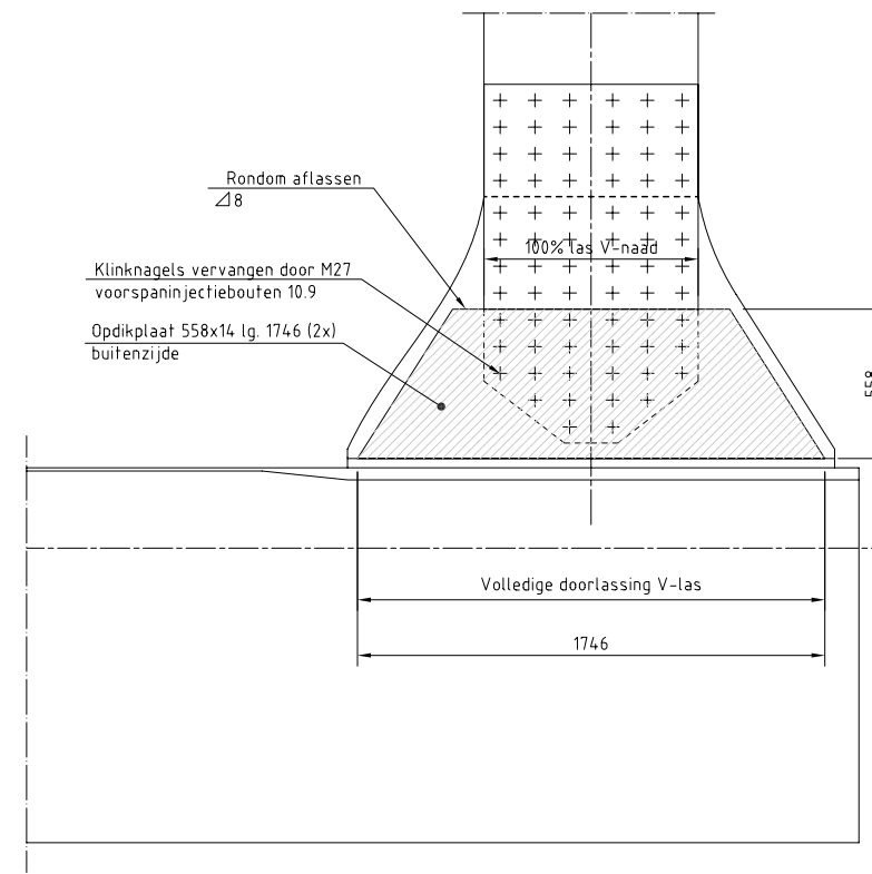
Detail versterking knoopplaat bij verticalen Schaal 1:20
