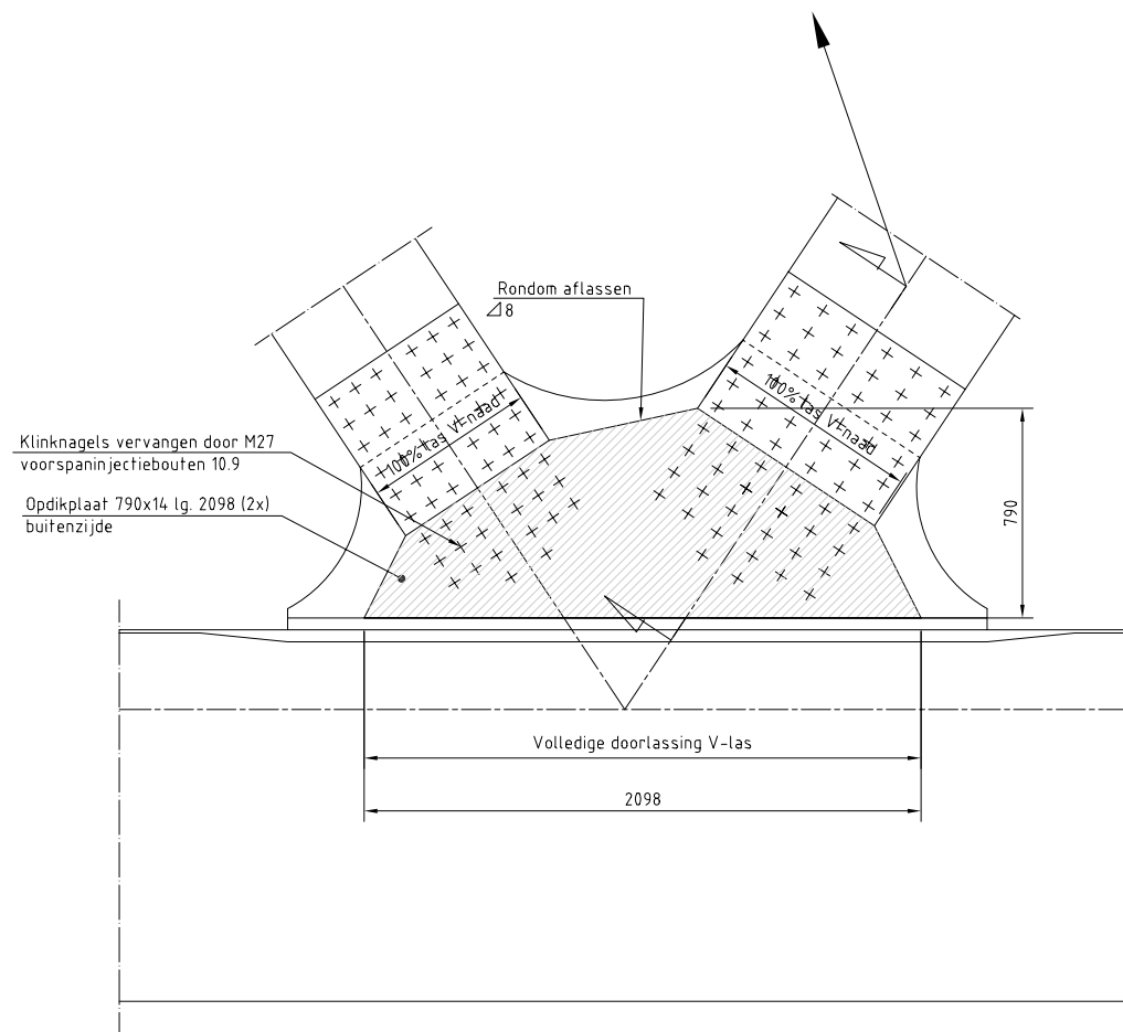
Detail versterking knoopplaat bij diagonalen Schaal 1:20
