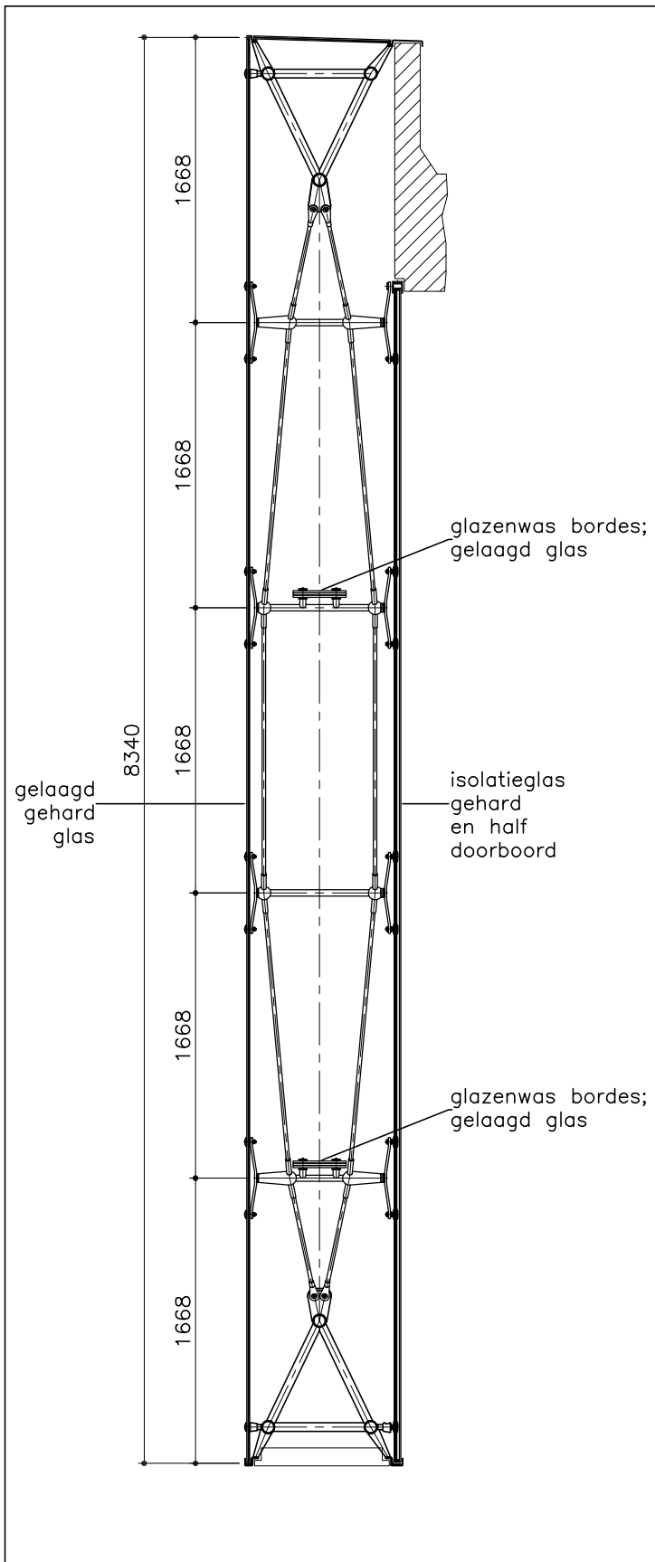
DOORSNEDE SPANT
