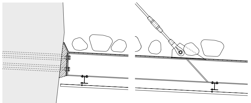
Détail ancrage et haubannage, échelle 1:50
