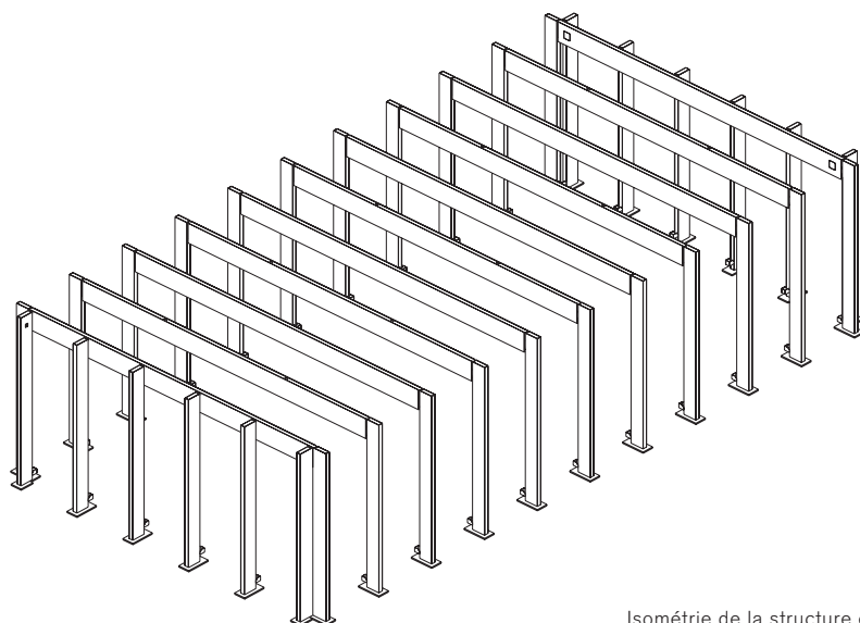
Isométrie de la structure en acier
